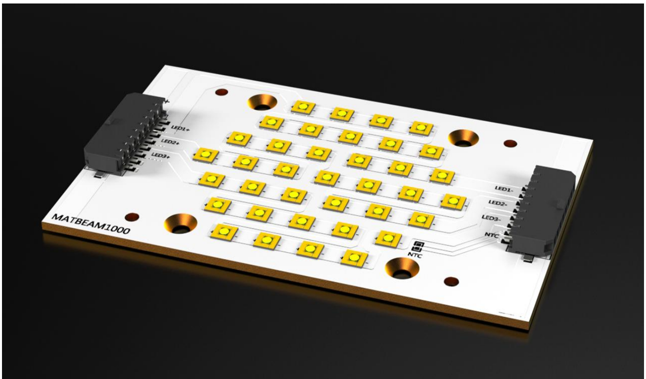
LED矩阵式光引擎光源板
