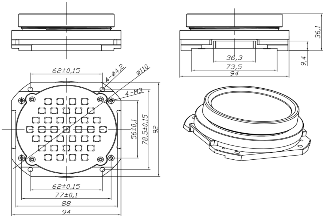
Toplite复眼模组光学镜头结构尺寸
